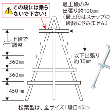
MBDSL型 仕様寸法図
