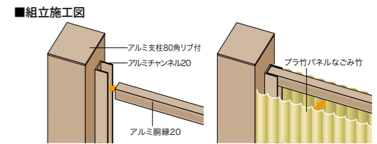
建仁寺垣なごみ 煤竹 両面 アルミ支柱80角リブ付ブラウン使用 基本セット
