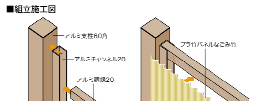
建仁寺垣なごみ イエロー 片面 アルミ支柱60角ブラウン使用 基本セット
