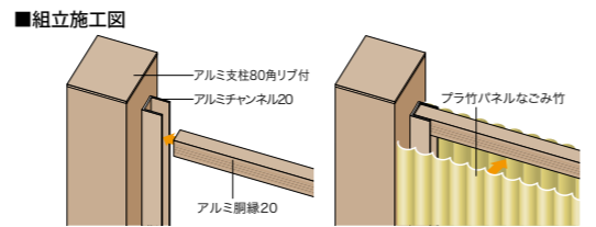
建仁寺垣なごみ イエロー 両面 アルミ支柱80角リブ付ブラウン使用 基本セット
