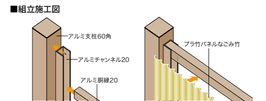
建仁寺垣なごみ 煤竹 片面 アルミ支柱60角ブラウン使用 基本セット
