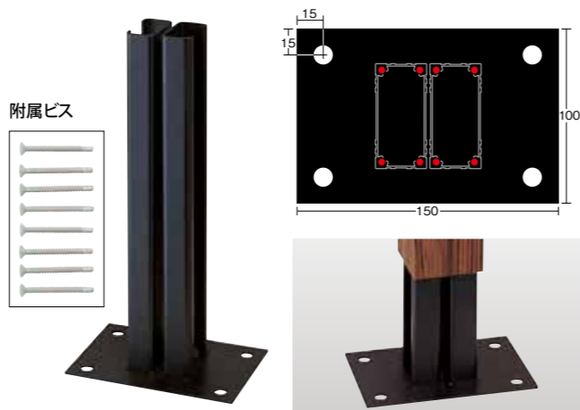
支柱サンロク角2本と組み合わせたところ
