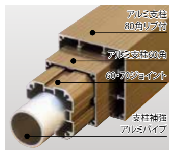
4層補強システム
