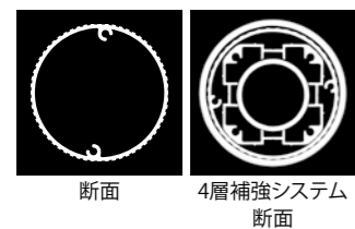
エイコーポール80φの中に組み込んだところ
