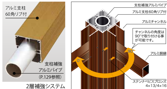
2層補強システム
