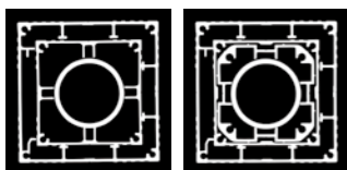
3層補強システム 断面 4層補強システム 断面
