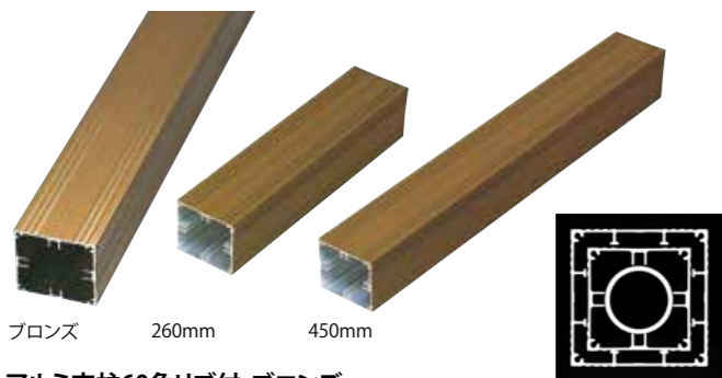
アルミ支柱60角リブ付 ブロンズ
