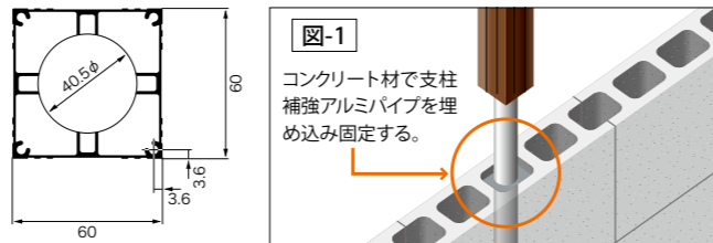
2層補強システム
