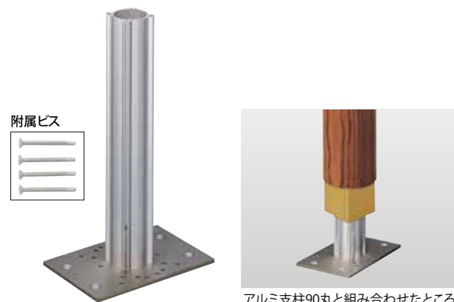
アルミ支柱90丸と組み合わせたところ
