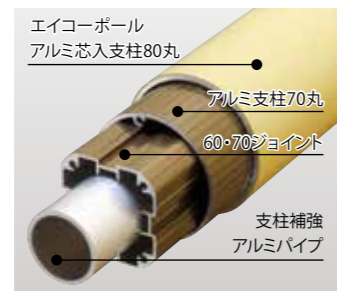
4層補強システム
