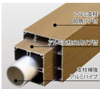
3層補強システム
