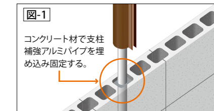
エイコーポール80φの中に組み込んだところ
