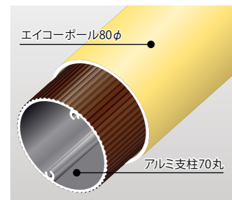
エイコーポール80φの中に組み込んだところ
