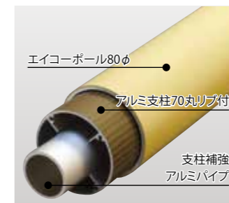
エイコーポール80φの中に組み込んだところ
