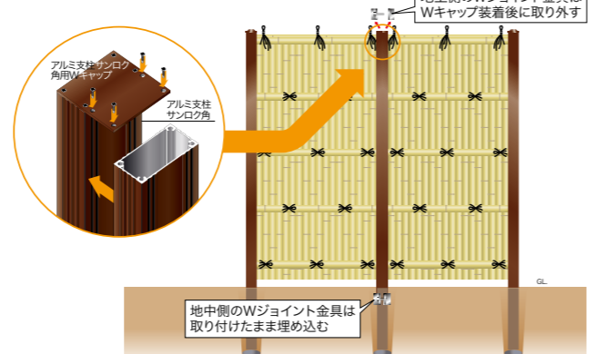
サンロク角 キャップW アルミ支柱 サンロク角
