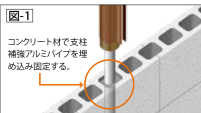
4層補強システム
