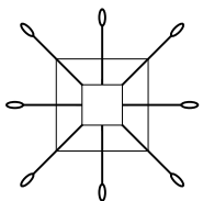
エイコーモッコタスキ 独立型 8点吊
