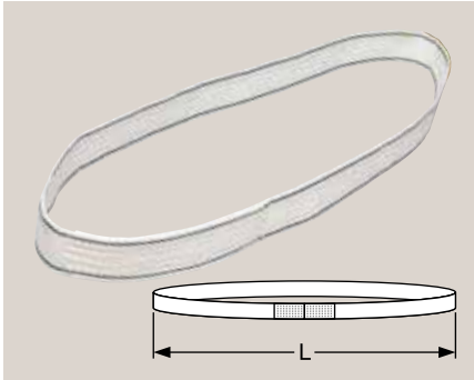
U-503 エイコーポリエステルベルトスリング REタイプ 白 1.6t用
