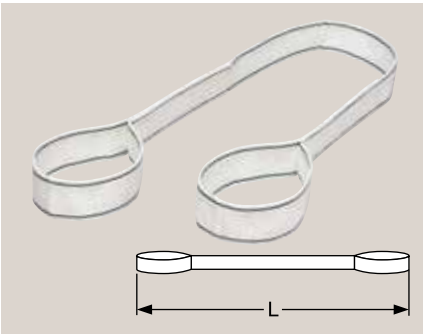
U-504 エイコーポリエステルベルトスリング BSタイプ 白 0.8t用
