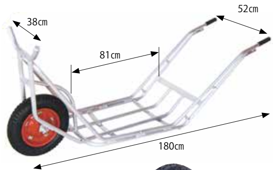
TR-2.50-4NA ノーパンクタイヤ
