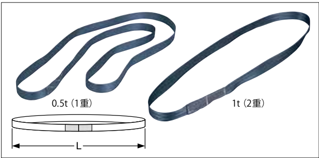
U-501 エイコーシートベルトスリング REタイプ
