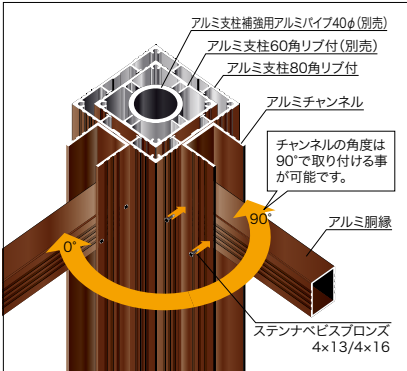
3層補強システム使用時
