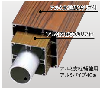
3層補強システム使用時
