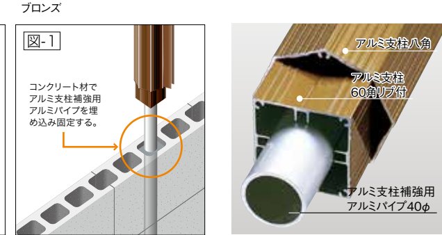
3層補強システム使用時
