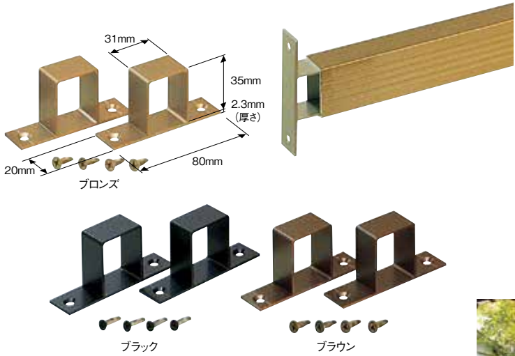
アルミ胴縁22ジョイントハット型
