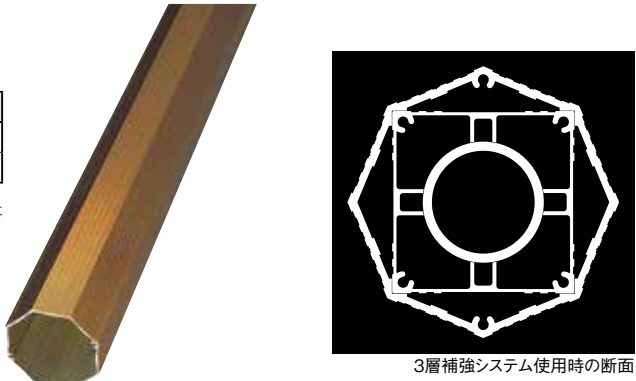
3層補強システム使用時の断面
