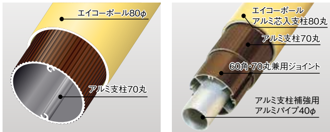
エイコーポール80φの中に組み込んだところ
