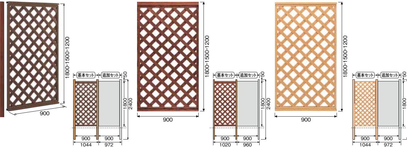
アルミ支柱70丸使用 (P.118参照)
