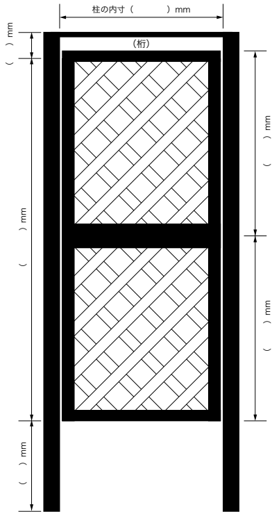
アルミ胴縁22タデミス枠使用 ラティス扉（B型）
