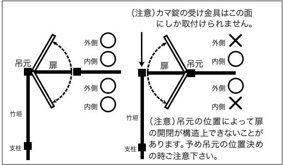
アルミ胴縁22タデミス枠使用 ラティス扉（A型）
