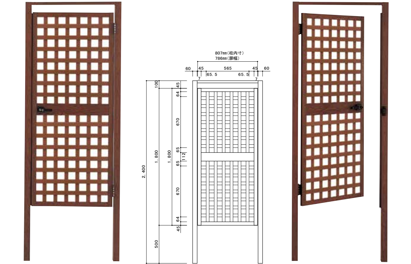
PAT-332 ラティス縦格子Ⅱ型扉セット1800(表)
