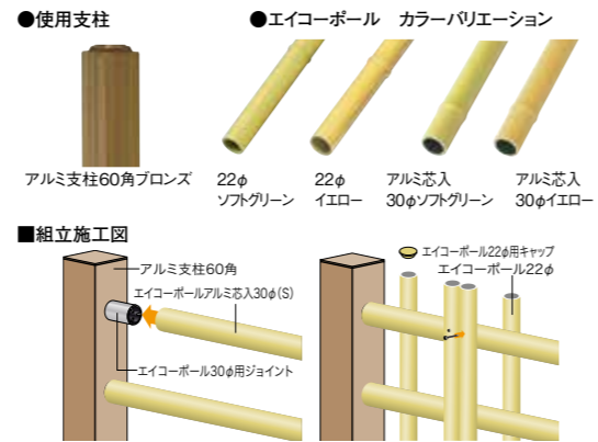
四つ目垣 900 アルミ支柱60角ブロンズ使用 基本セット(両柱) ソフトグリーン・イエロー
