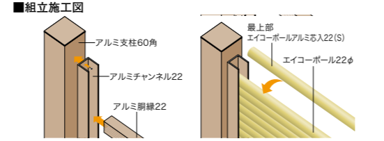
御簾垣22 アルミ支柱60角ブロンズ使用 基本セット(両柱) ソフトグリーン・イエロー
