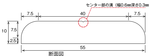
ダークブラウン ナチュラルブラウン オーク 断面図の写真
