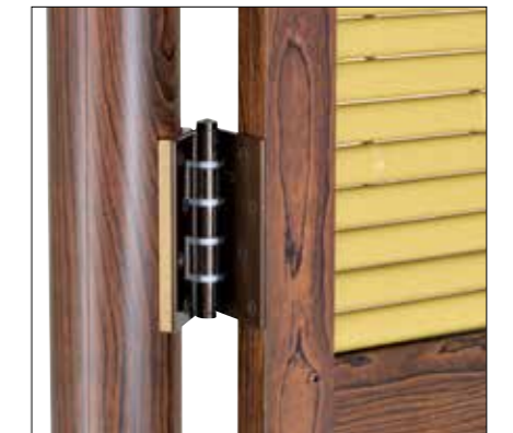
丸柱用蝶番取付板+扉用大型ステンレス蝶番による取付方法
