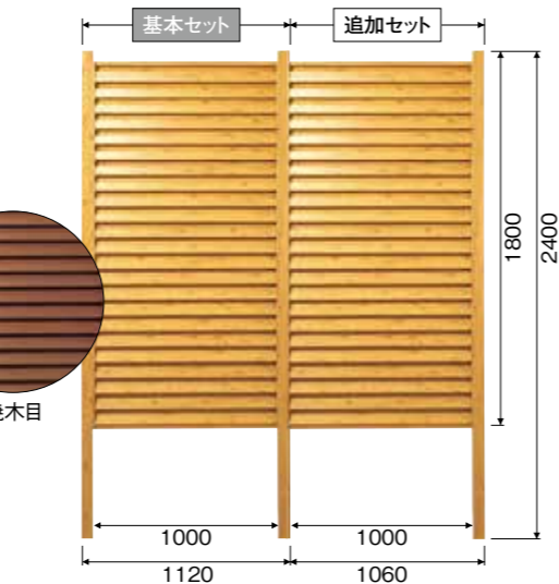
PU-417 アルミボードルーバー60角 オーク木目 W1120×H1800mm 基本セット【両柱付】 ¥151,880
