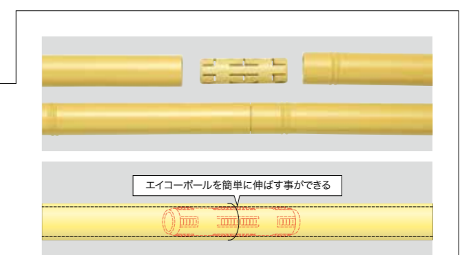
高耐候AS系 アイコーポール連結用ジョイント
