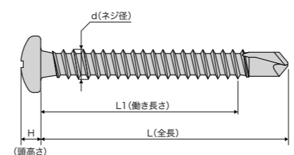
ナベ型ビス寸法表示
