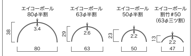
●エイコーポール半割竹断面図
