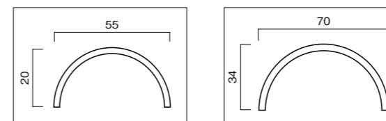
エイコープラ横竹#55 エイコープラ笠竹#70
