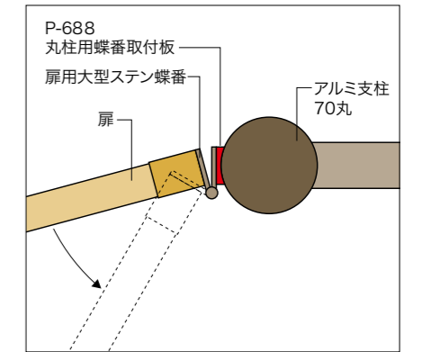
丸柱用蝶番取付板+扉用大型ステンレス蝶番による取付方法
