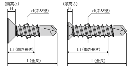
サラ型ビス寸法表示
