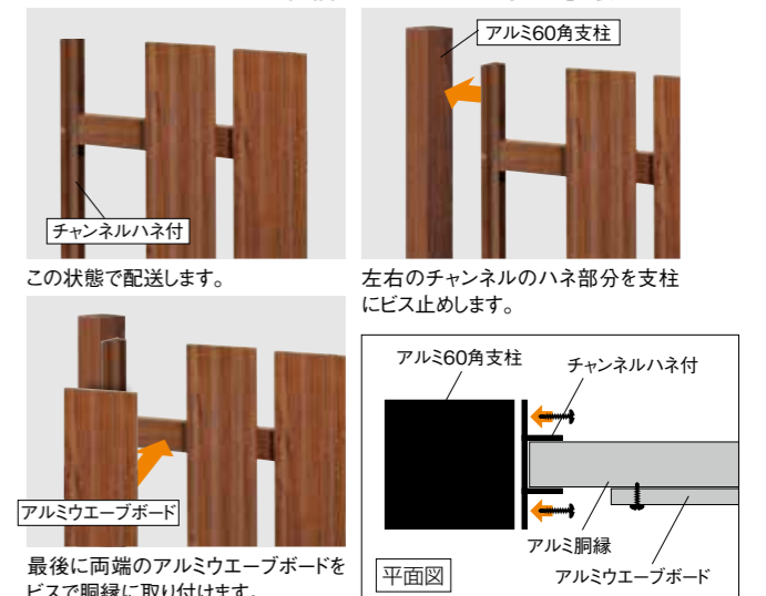
アルミウエーブボード柵II型ユニット (黒木目・焼木目・オーク木目)
