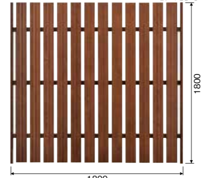
アルミウエーブボード柵II型ユニット (黒木目・焼木目・オーク木目)
