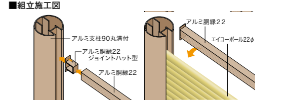
御簾垣I型 アルミ支柱90丸溝付ブロンズ使用 基本セット(両柱) ソフトグリーン・イエロー
