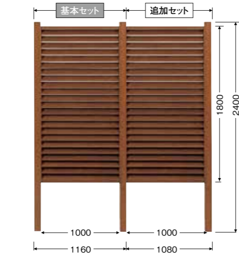
PU-421 アルミボードルーバー80角 焼木目 W1160×H1800mm 基本セット【両柱付】 ¥172,120
