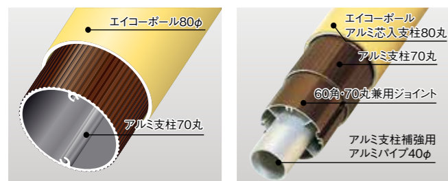
エイコーボール80φの中に組み込んだところ
