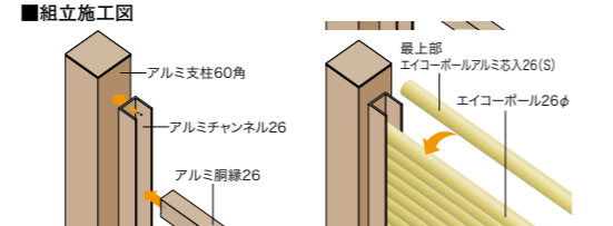
御簾垣26 アルミ支柱60角ブロンズ使用 基本セット(両柱) ソフトグリーン・イエロー
