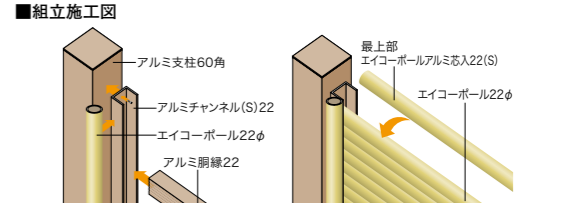
御簾垣II型 アルミ支柱60角ブロンズ使用 基本セット(両柱) ソフトグリーン・イエロー
