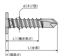
特平頭型ビス寸法表示
