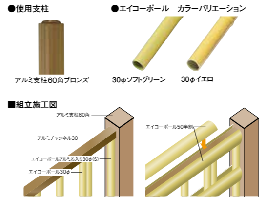
金閣寺垣 610 アルミ支柱60角ブロンズ使用 基本セット(両柱) ソフトグリーン・イエロー
