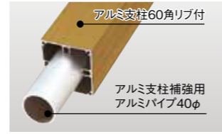
2層補強システム使用時
