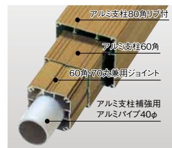
4層補強システム使用時
