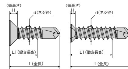
サラ型ビス寸法表示
