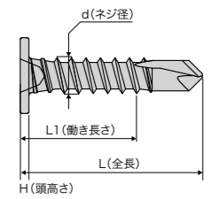
特平頭型ビス寸法表示
