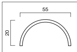
エイコープラ横竹#55
