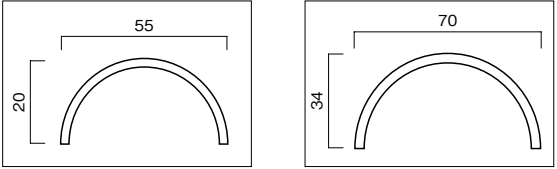
エイコープラ横竹#55
