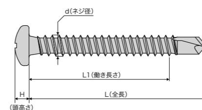
ナベ型ビス寸法表示
