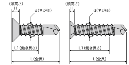
サラ型ビス寸法表示
