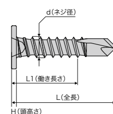
特平頭型ビス寸法表示
