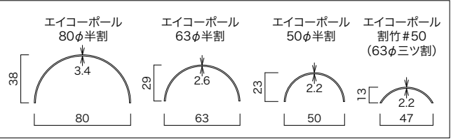
●エイコーポール半割竹断面図
